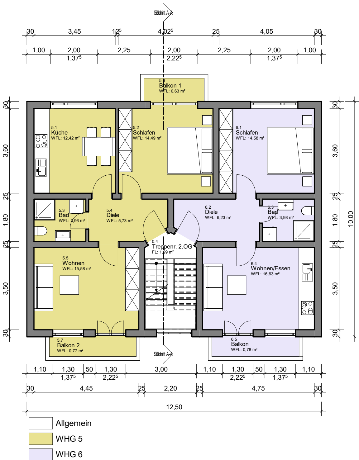
Grundriss 2. Obergeschoss M 1 : 100
